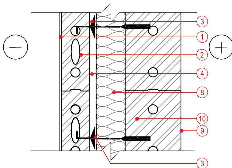
PJŪVIS 1-1
